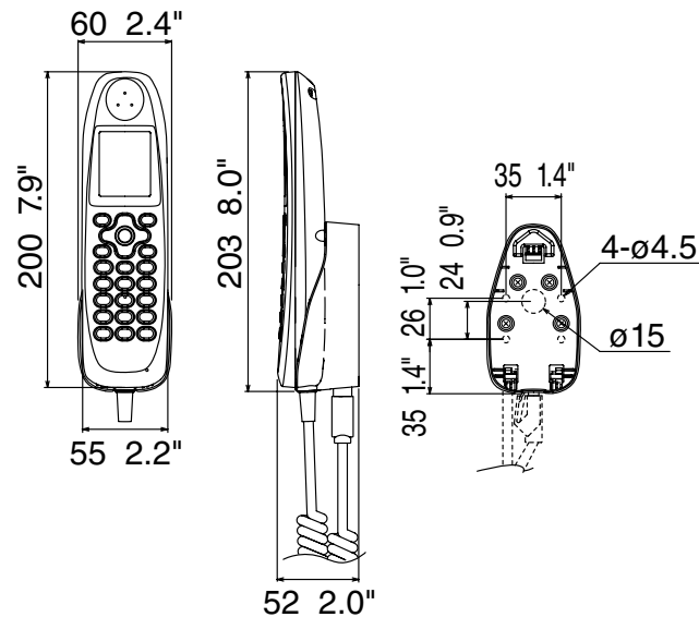
FELCOM250/500 Handset FB-8000
