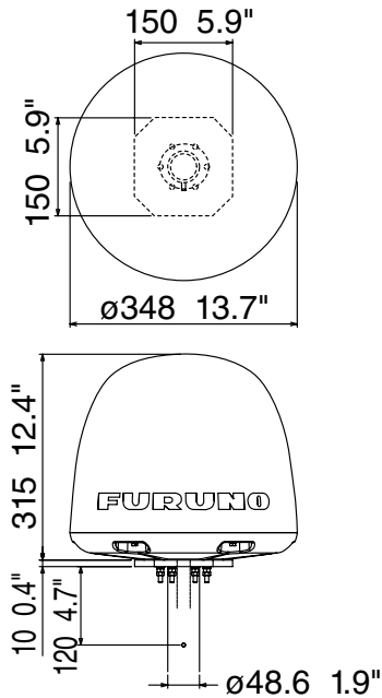
FELCOM250 Antenna FB-1250
