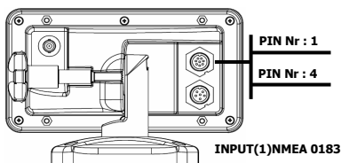
Voeding / Data kabel
