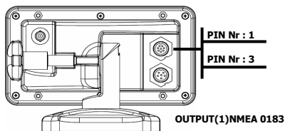
Voeding / Data kabel
